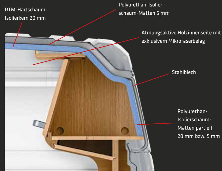
Malibu Van: aufwendige Karosserie-Isolationsmaßnahmen
